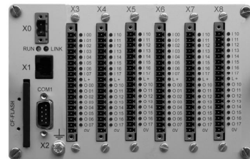
ICS-Gehäuse mit Frontplatte, Rückwand und Zubehör. 7 Leiterplatten-Steckplätze
