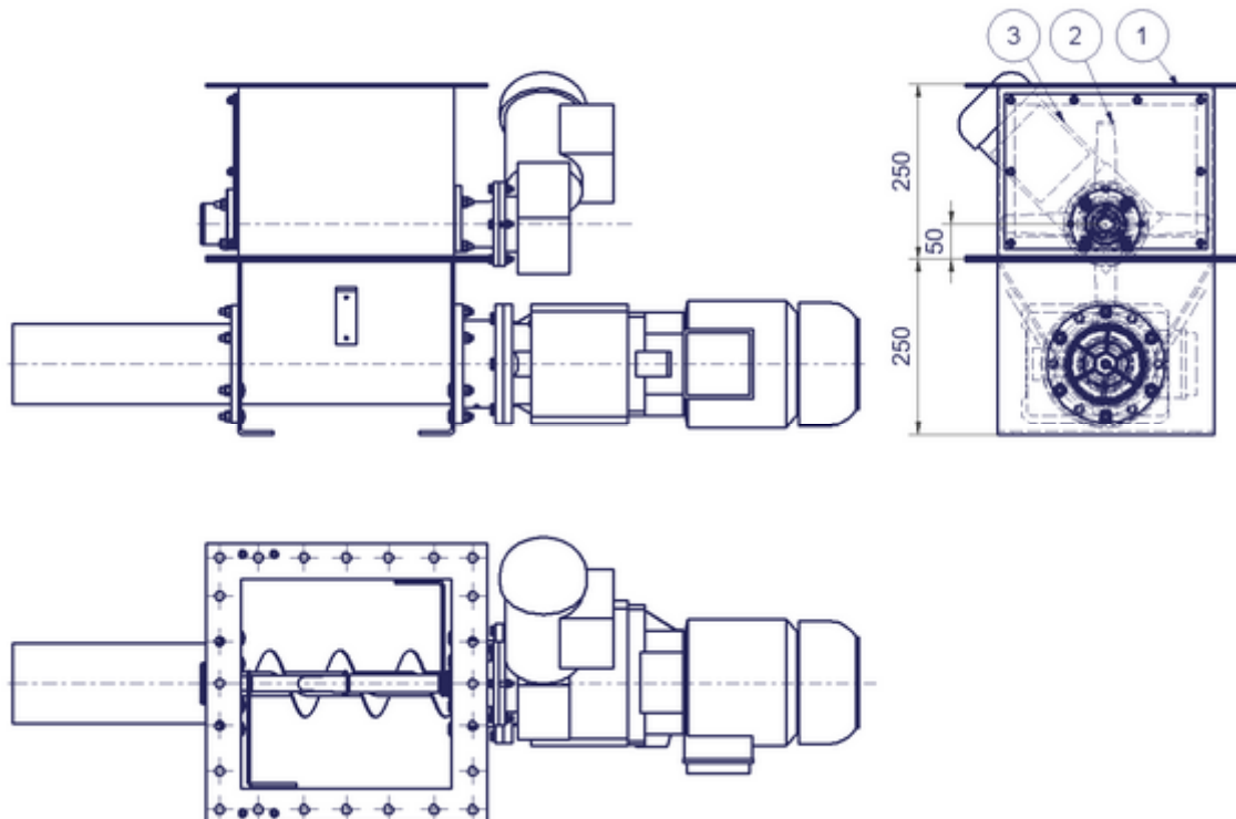
Abbildung DS21-100 mit Option Rührwerksaufsatz (Bauhöhe 250 mm, gleiche Anschlussflansch)
